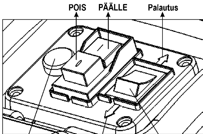
Palautusnappi (moottorinsuo ja) Veto Kierrossuunnankytkin
